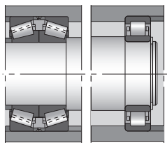
图5 配组圆锥滚子轴承—圆柱滚子轴承
