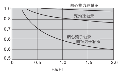
图3：根据轴承负荷修正极限转速
