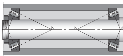
图11 圆锥滚子轴承 O型配置
