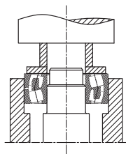
图5 内外圈均为紧配合
