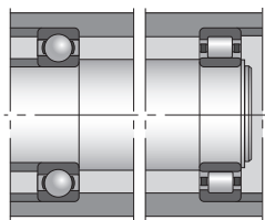
图2 深沟球轴承—圆柱滚子轴承
