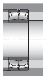
图15 双列调心滚子轴承
