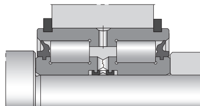
图19 SL系列轴承
