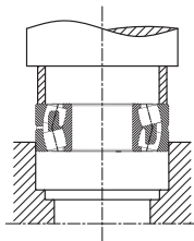
图4 外圈紧配合
