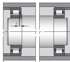
图14 圆柱滚子轴承
