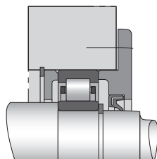
图22 圆柱滚子轴承
