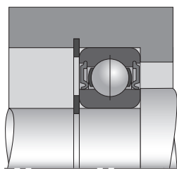
图16 深沟球轴承
