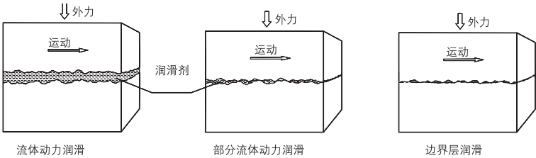
图：润滑机理
