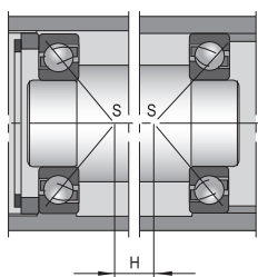
图9 角接触球轴承 X型配置
