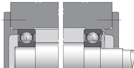
图23 通过波形弹簧片预紧的深沟球轴承
