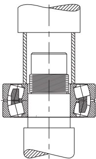
图3 内圈紧配合
