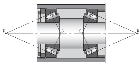
图10 圆锥滚子轴承 X型配置
