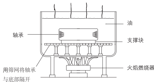
图2 油池加热
