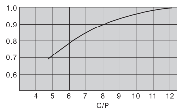
图4：合成负荷下极限转速的修正
