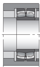
图20 双列调心滚子轴承
