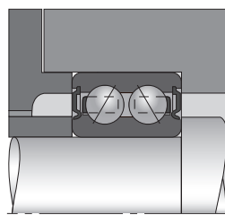
图17 双列角接触球轴承
