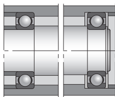
图1 深沟球轴承—深沟球轴承
