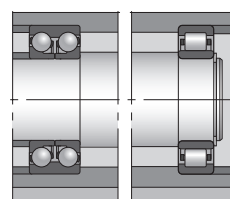
图4 双列角接触球轴承—圆柱滚子轴承
