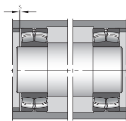
图13 双列调心滚子轴承
