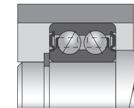
图21 双列角接触球轴承
