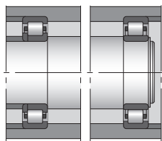
图3 圆柱滚子轴承—圆柱滚子轴承
