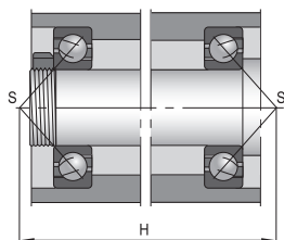
图8 角接触球轴承 O型配置
