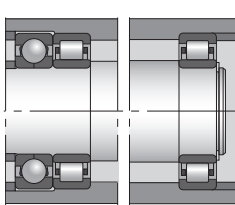
图6 组合轴承—圆柱滚子轴承
